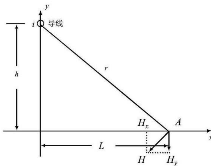
图 3.1-4 磁场向量图
