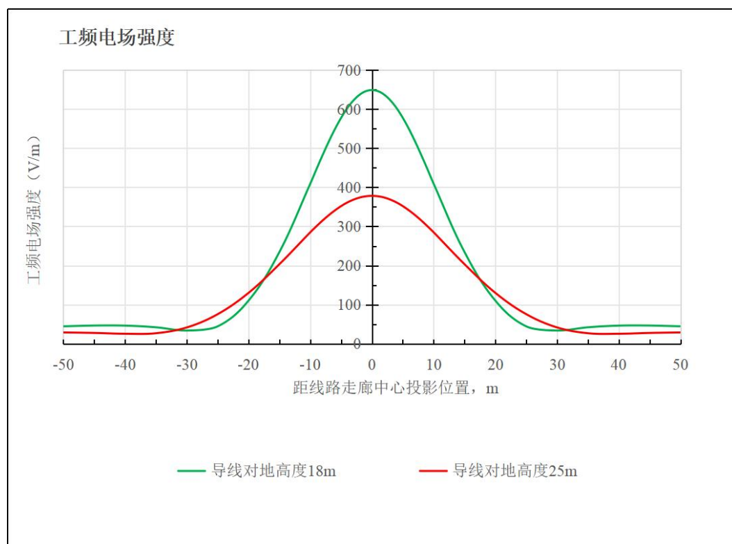
图 3.1-7 重新紧放线 110kV 同塔双回架空输电线路下方距地面 1.5m 高度处工频电场强度预测结果趋势图
