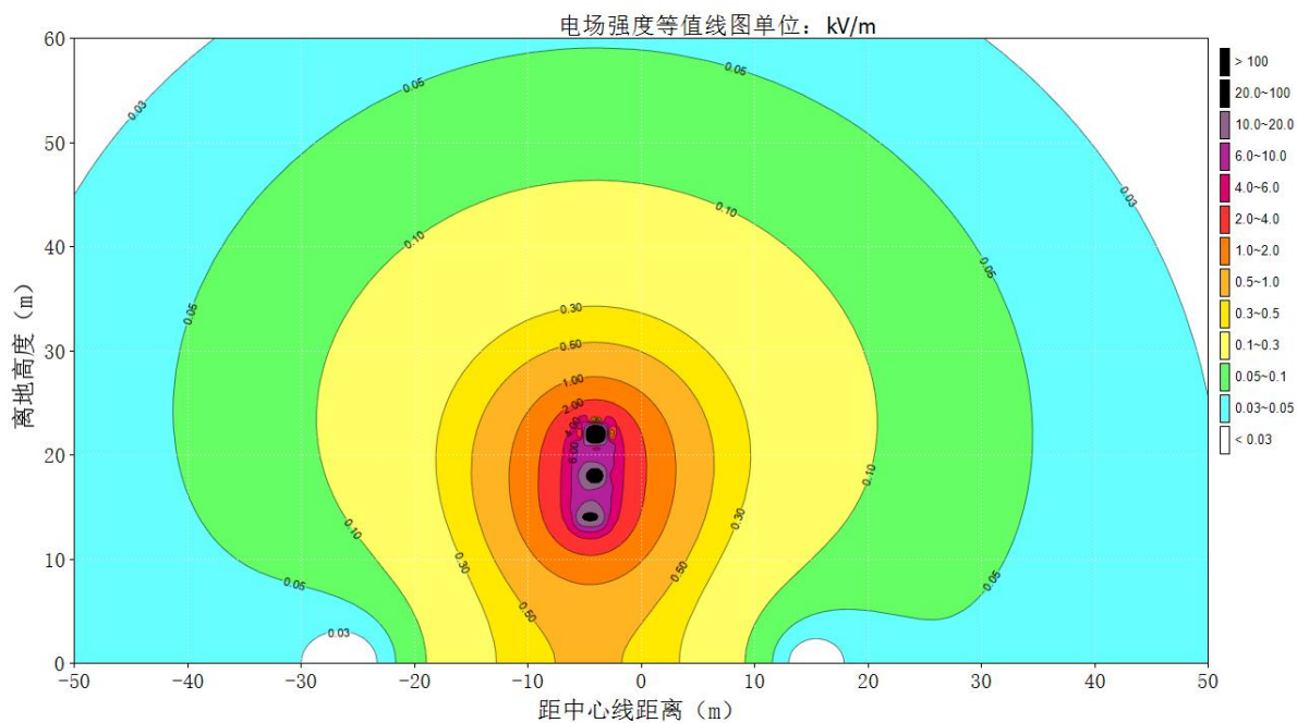
图 3.1-13 新建单回架空（双设单挂）输电线路周围工频电场强度等值线图（导线对地高度 14m）
