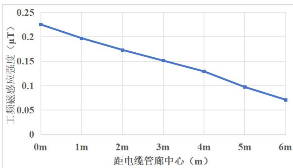
图3.2-2 类比断面工频磁感应强度的变化趋势图
