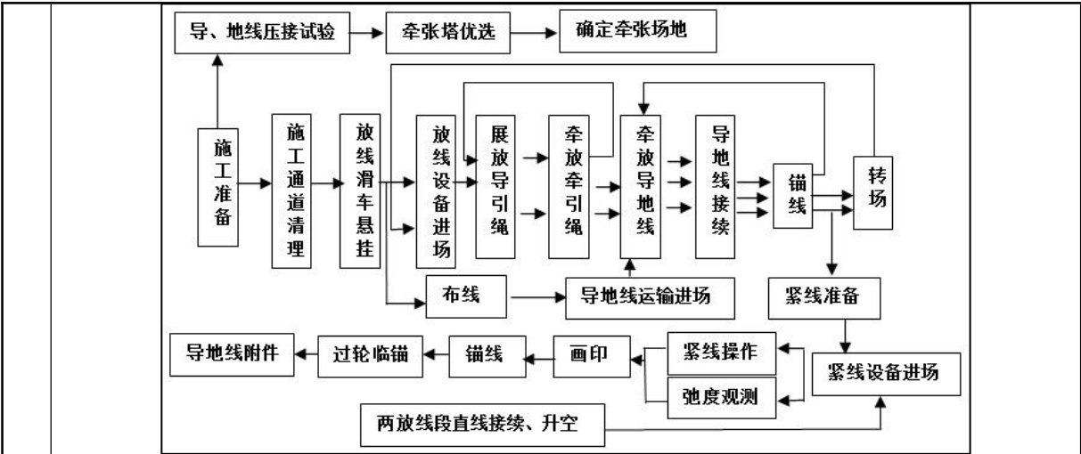
图 2 架线施工流程图
