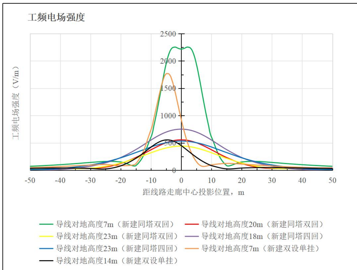
图 3.1-5 新建 110kV 同塔双回架空线路、新建同塔四回架空线路、新建 110kV 单回架空（双设单挂）输电线路下方距地面 1.5m 高度处工频电场强度预测结果趋势图
