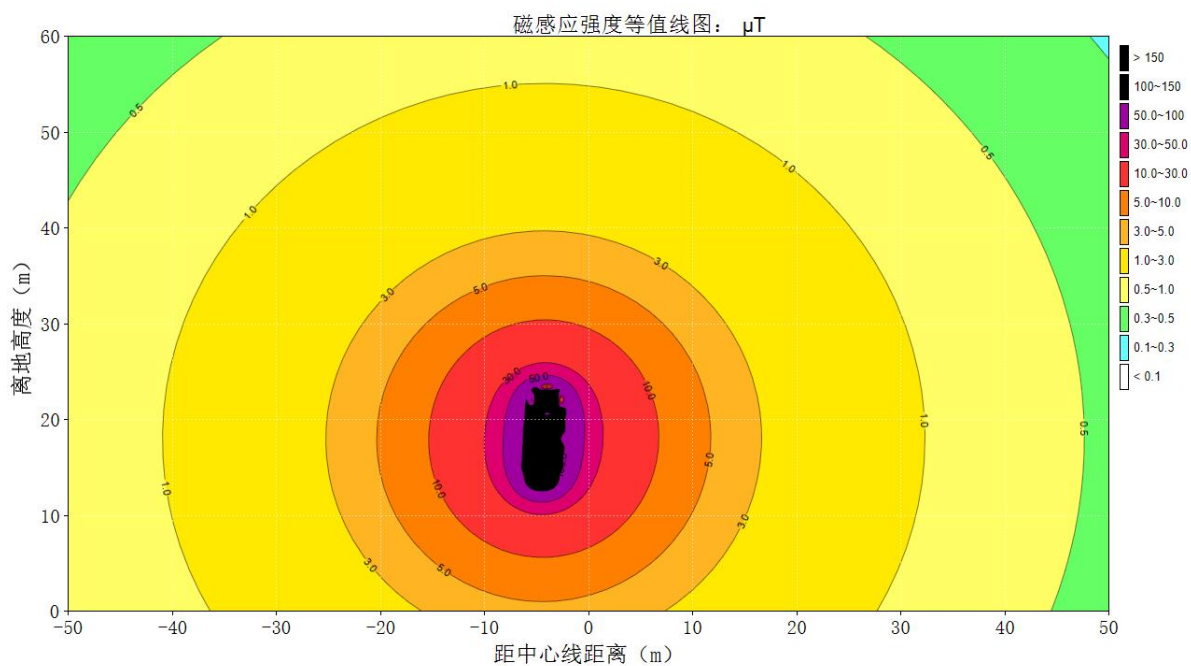
图 3.1-14 新建单回架空（双设单挂）输电线路周围工频磁感应强度等值线图（导线对地高度 14m）
