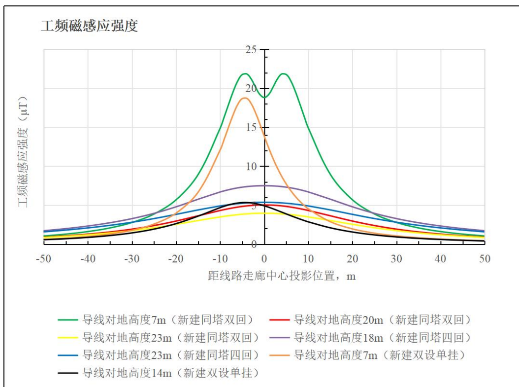
图 3.1-6 新建 110kV 同塔双回架空线路、新建同塔四回架空线路、新建 110kV 单回架空 (双设单挂) 输电线路下方距地面 1.5m 高度处工频磁感应强度预测结果趋势图
