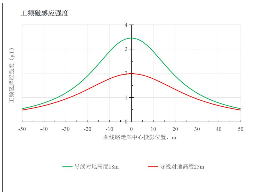
图 3.1-8 重新紧放线 110kV 同塔双回架空输电线路下方距地面 1.5m 高度处工频磁感应强度预测结果趋势图
