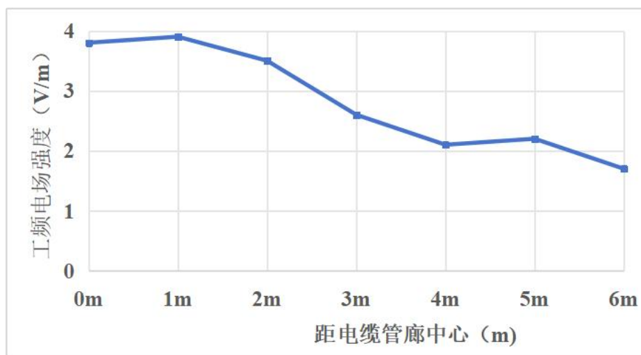
图3.2-1 类比断面工频电场强度的变化趋势图
