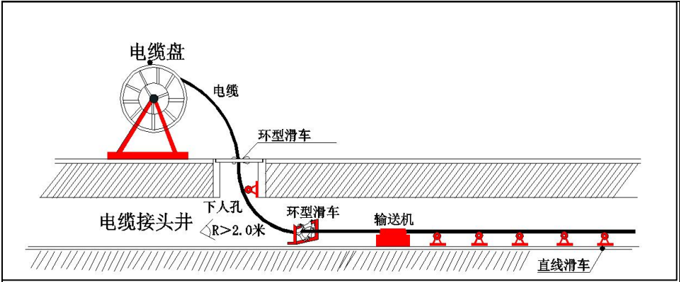
图 3 电缆敷设示意图
