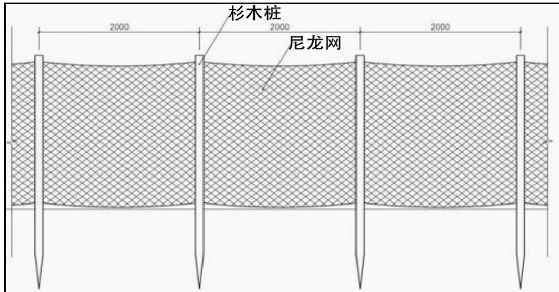
图2-5 红树林养护断面图
