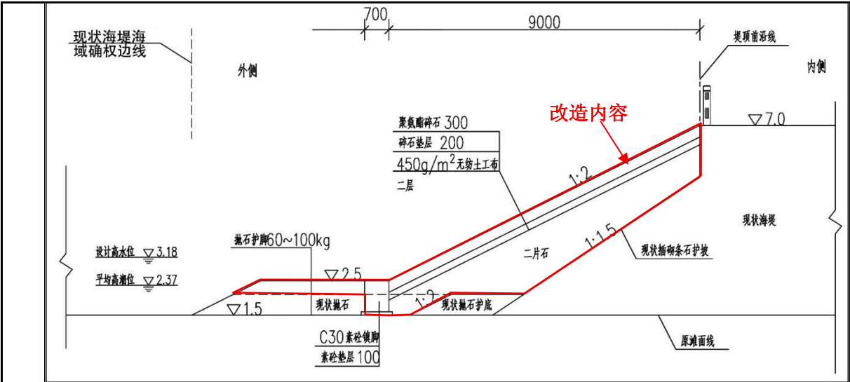
图 2-9 海堤生态化典型断面图
