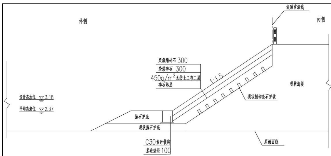
图 2-3 《泉州市晋江市深沪湾海洋生态保护修复项目实施方案》海堤断面图
