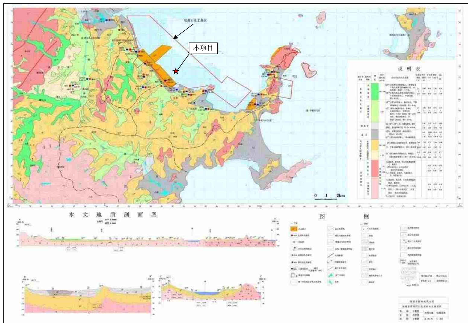
图 5.3-1 评价区域地质地貌图
