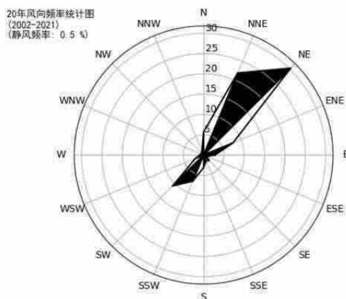
图 5.2-2 崇武风向玫瑰图 (静风频率 0.5%)
