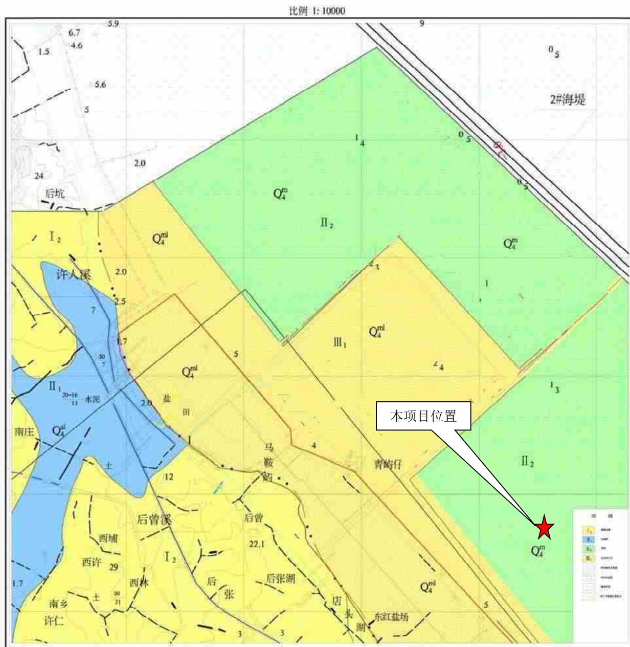
图 5.3-2 场地所在区域地质地貌图
