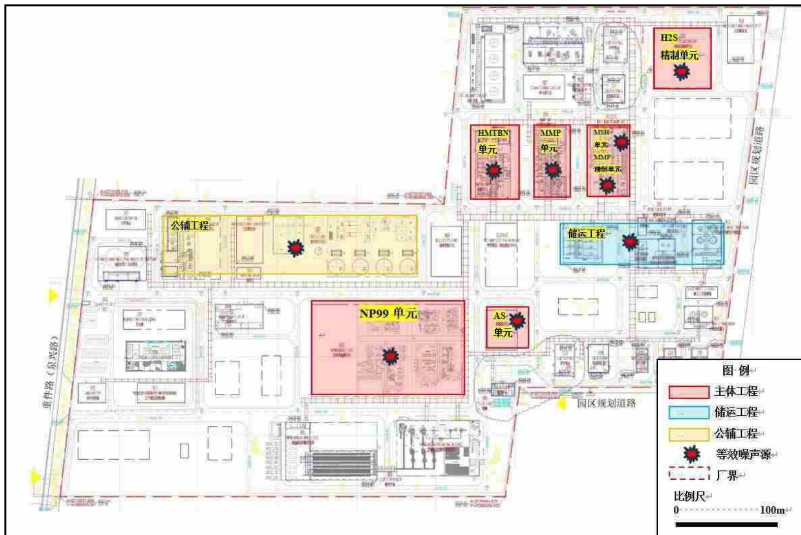
图 5.4-1 本项目新增噪声污染源运营期噪声平面布置图
