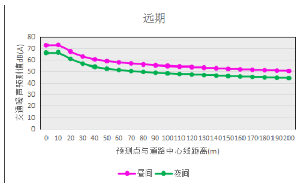
图 8-1 二号路交通噪声预测衰减分布图
