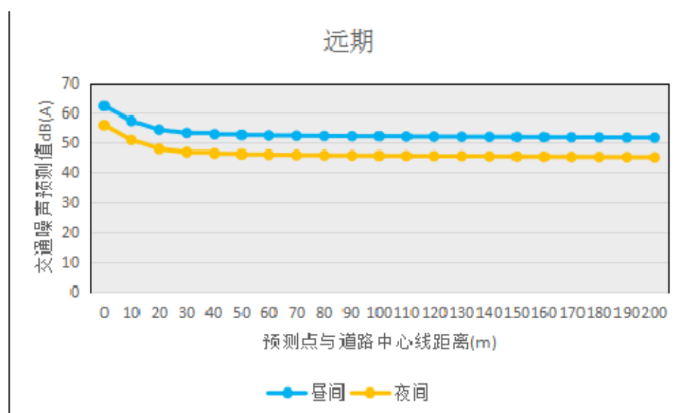
图 8-1 鞋纺二路交通噪声预测衰减分布图
